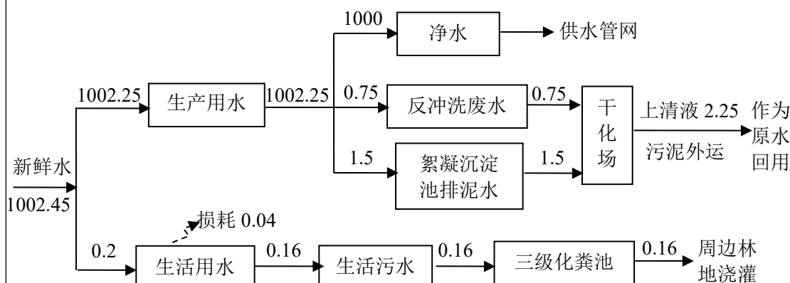
图 4-1 水平衡图 (单位: t/d)
