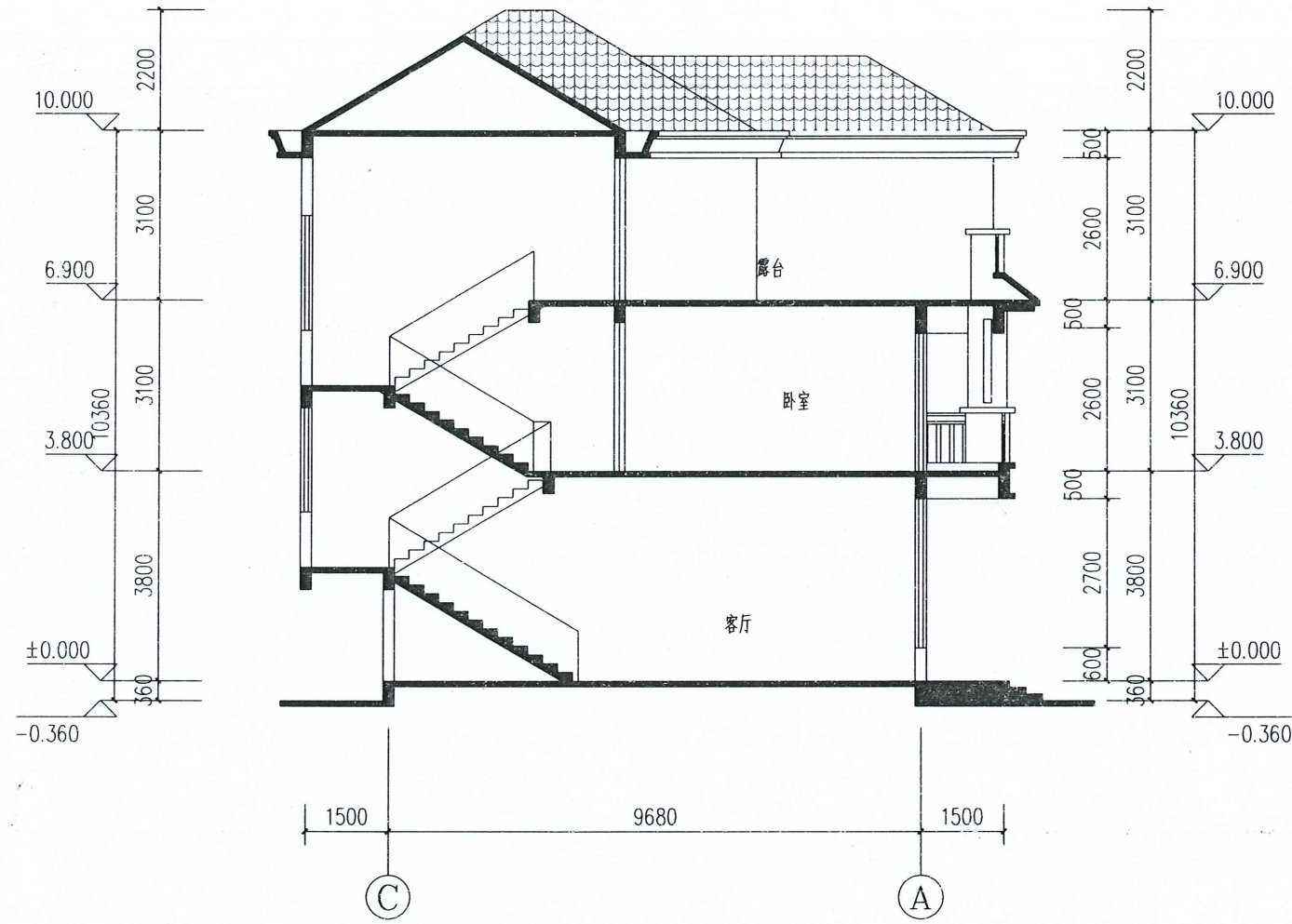
剖面图 1:100
