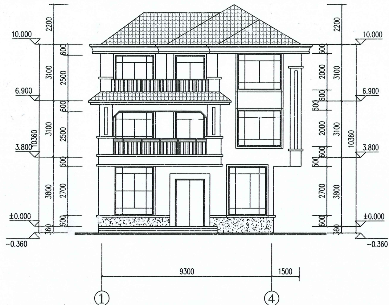
①-④立面图 1:100
