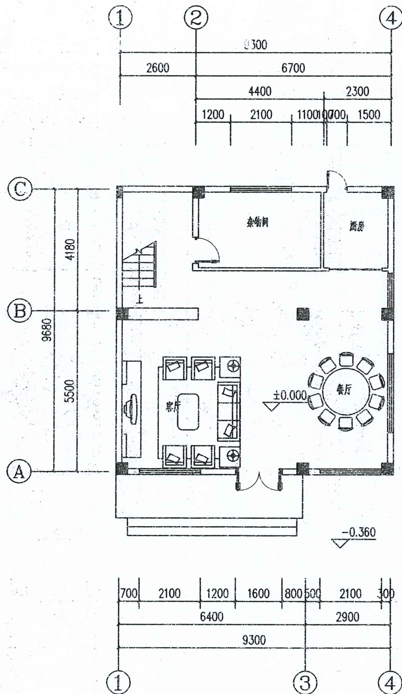
一层平面图 1:100
