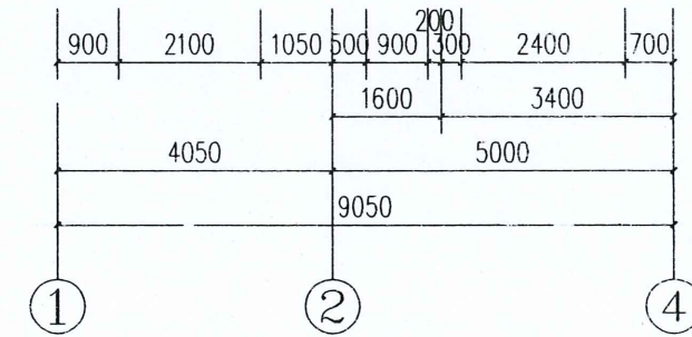
二三层平面图 1:100
