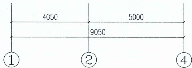
坡屋顶平面图 1:100
